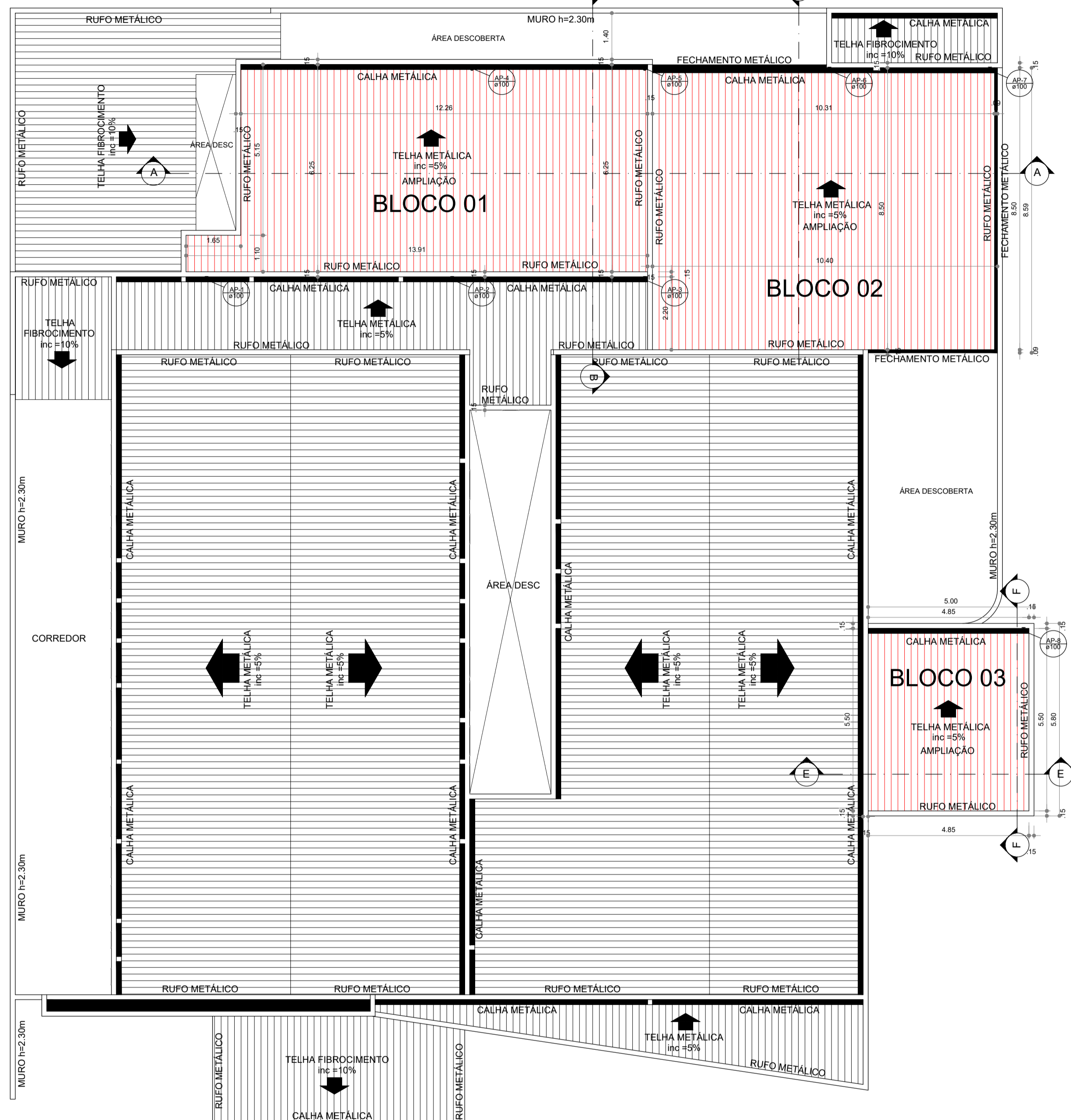
2 PLANTA DE COBERTURA Esc. 1:100
